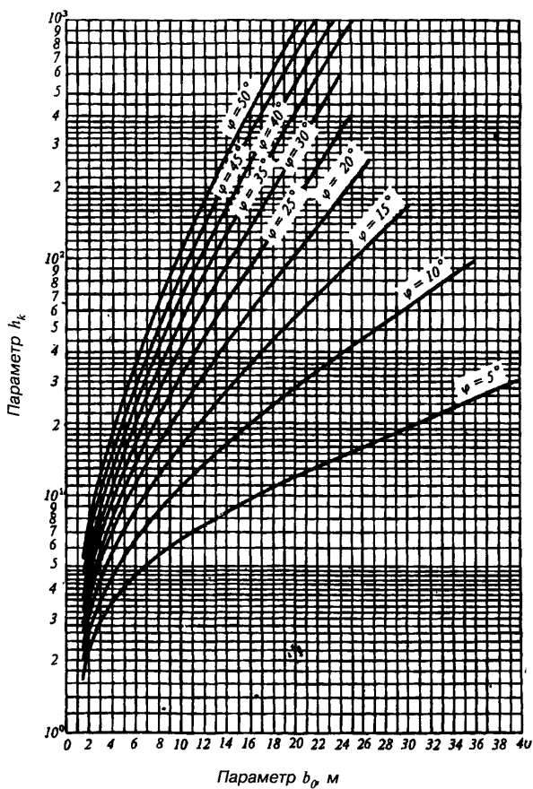
Черт. 6. Графики для определения параметра b_0
