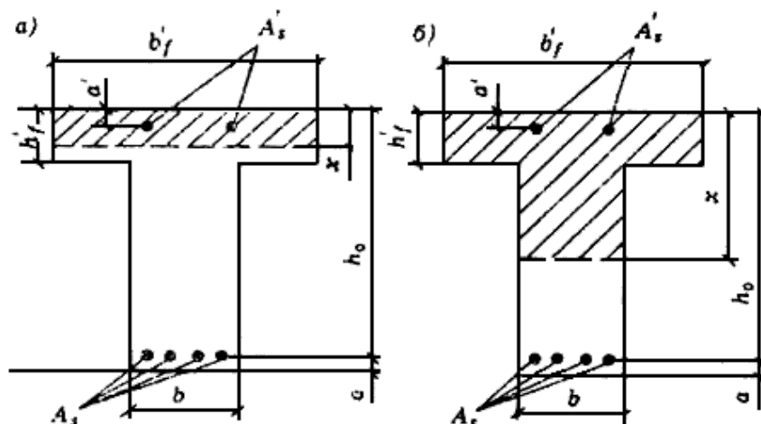
Черт.5. Положение границы сжатой зоны в сечении изгибаемого железобетонного элемента \alpha - в полке; \beta - в ребре
